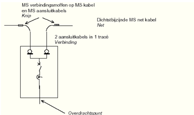
Figuur 4 Zuivere MS aansluiting (0,3 – 3 MVA)
