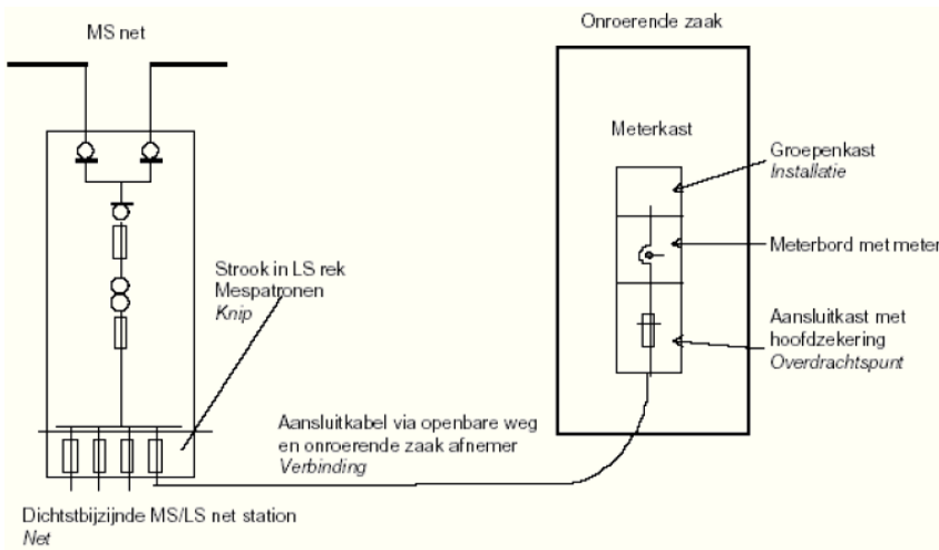
Figuur 3 LS aansluiting af LS-rek transformator (60 – 300 kVA)
